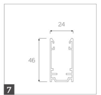
Profilo laterale
